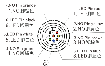
8線三色腳位
