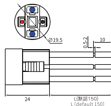
專用接插件 Connector
