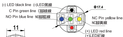
鍍金/鍍銀引腳 Pin
