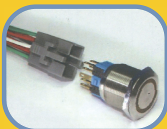
連接示意圖
