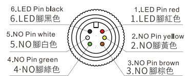
6線單色腳位
