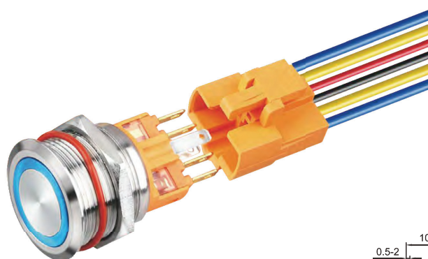
加粗觸點，通過電流更大 Big Contact
