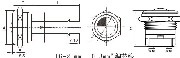
16~25mm 0.3mm 2 銅芯線 Copper core wire
