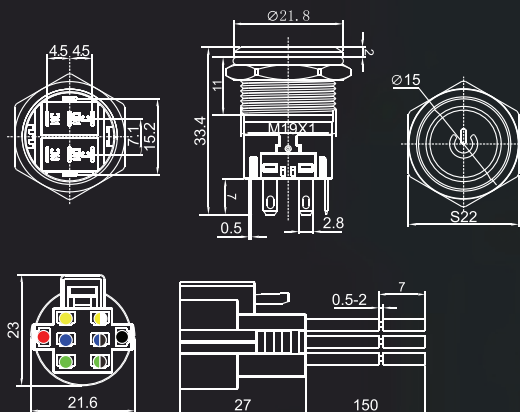
可做2常開2常閉 2NO2NC
