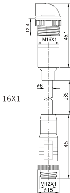
帶燈, 大旋柄 LED, Big Handle
