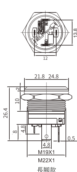
無極LED燈珠，大觸點 Non-Polar LED
