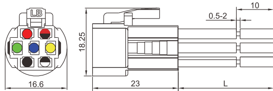
16M4 專用接插件 Connector
