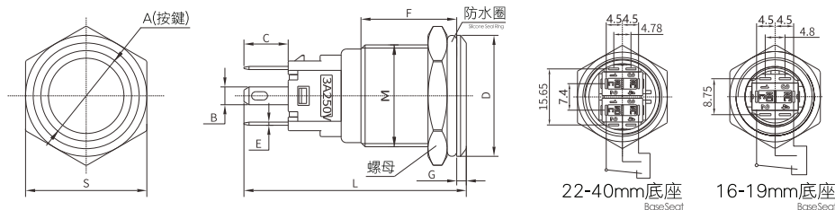
配套專用插件 Connector
