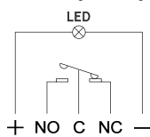
3檔 原理圖 Schematic diagram of 3 gear
