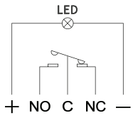
3檔 原理圖 Schematic diagram of 3 gear
