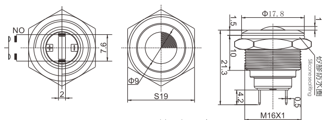
PBM16E外型尺寸 Outline Dimension
