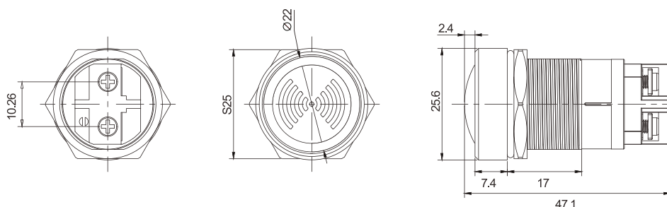
304金屬面罩，IP65 304StainlessSteel · IP65
