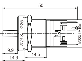
專用插件，防誤碰設計 Connector
